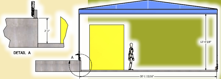
Séchoir à bois et autre matériaux
